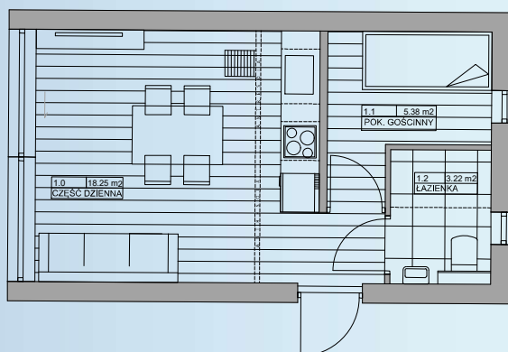
RZUT PARTERU
